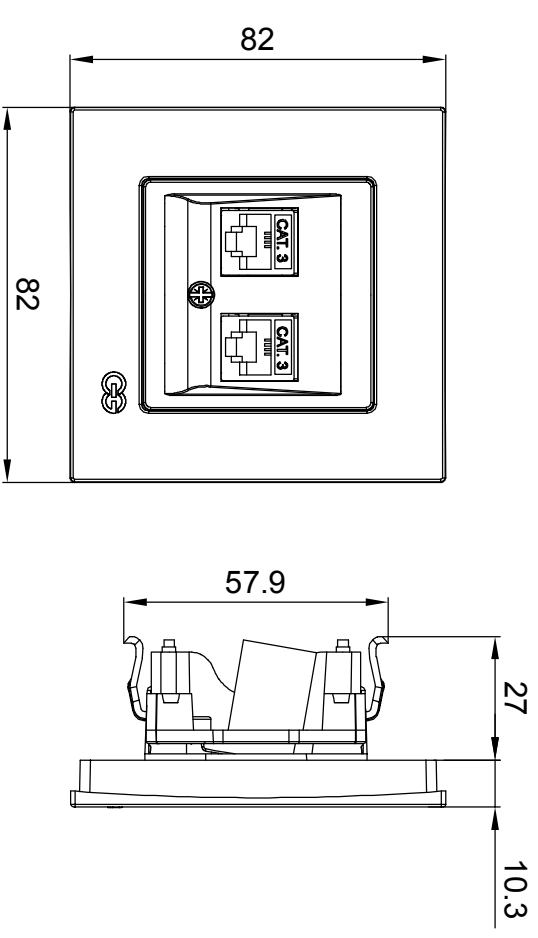
Ürün Boyutları / Product Dimensions
