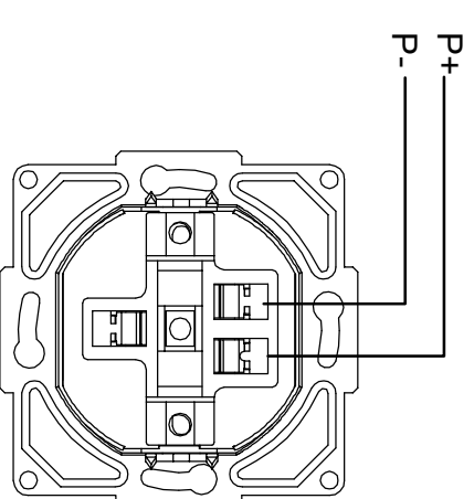
Bağlantı Şeması / Wiring Diagram
