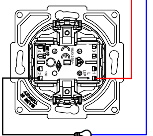
Bağlantı Şeması / Wiring Diagram
